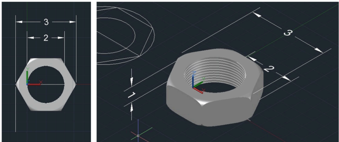
Gambar 3.4 Autocad Mur
