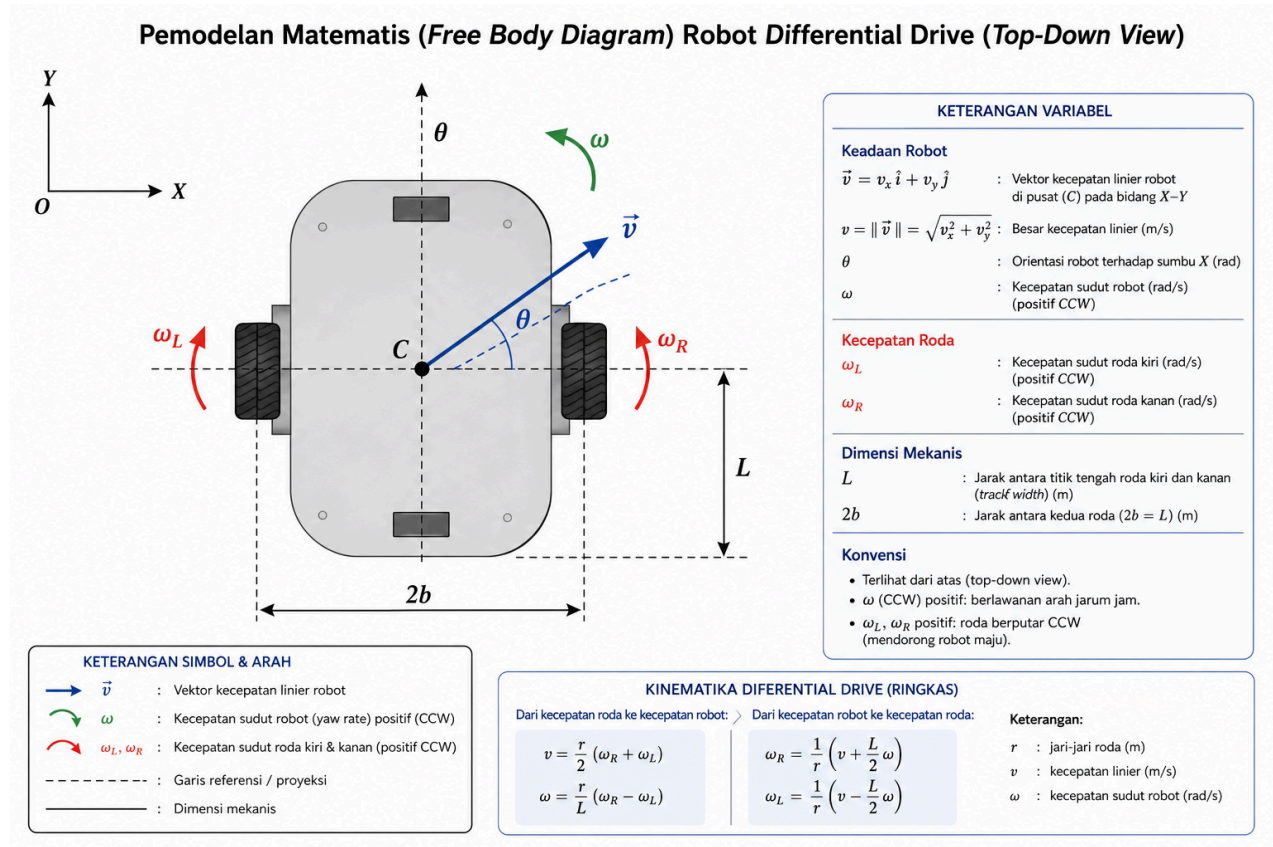
Gambar 4.2 Pemodelan Matematis Struktur Robot
